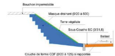
Coupe type d'une infrastructure en déblai avec masque drainant
