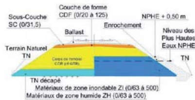
Coupe type d'une Infrastructure en remblai
