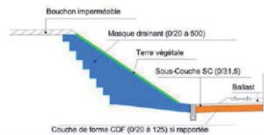
Coupe type d'une infrastructure en déblai avec masque drainant
