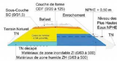
Coupe type d'une infrastructure en remblai
